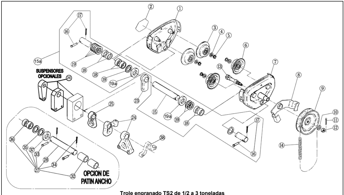
Trole engranado TS2 de 1/2 a 3 toneladas
