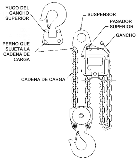
Figura 3-223 Instalación de la suspensión en los polipastos/tecles de caída doble TCR/S/L1000P, TCR2000P2, TCR/K/L6000P2
