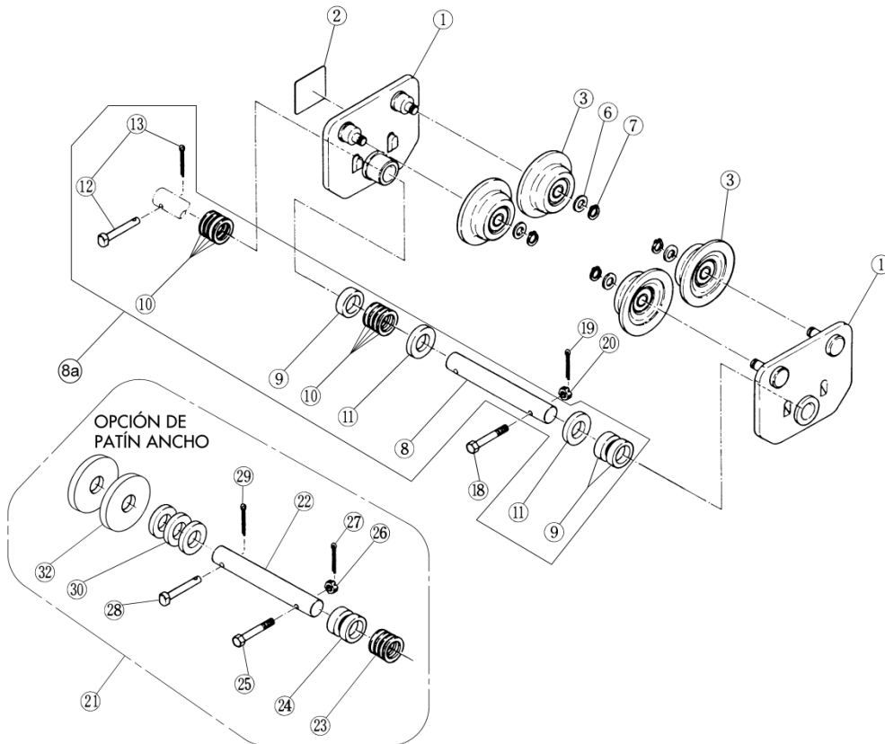
Trole de empuje de 5 toneladas Figura 8-1 Trole de empuje TF2
