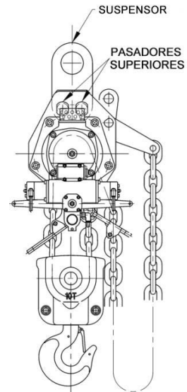
Figura 3-24 Instalación de la suspensión en TCR10000P2
