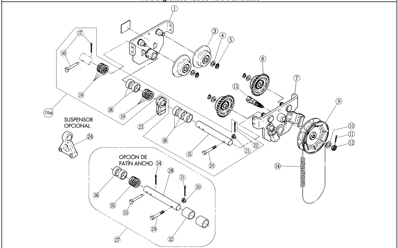
Trole engranado TS2 de 5 toneladas
