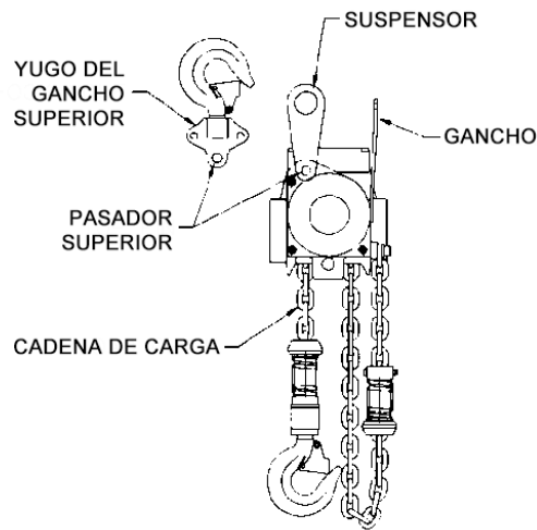
Figura 3-212 Instalación de la suspensión en los polipastos/tecles de una caída TCR/S/L250P, 500P, 3000P y TCK3000
