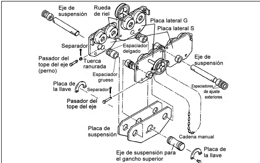
Figura 3-297 Ensamblaje del trole - Capacidades de 15 a 20 toneladas (manual)
