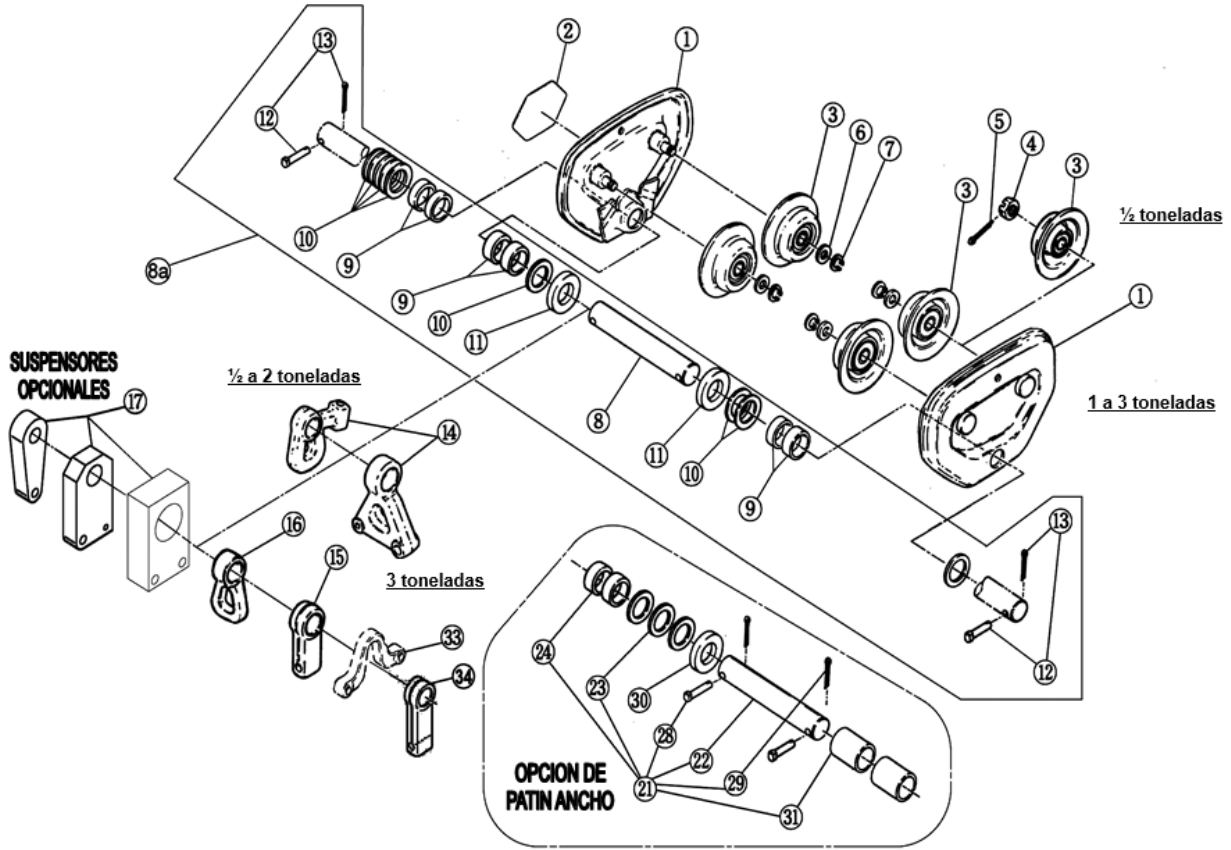
Trole de empuje TF2 de 1/2 a 3 toneladas
