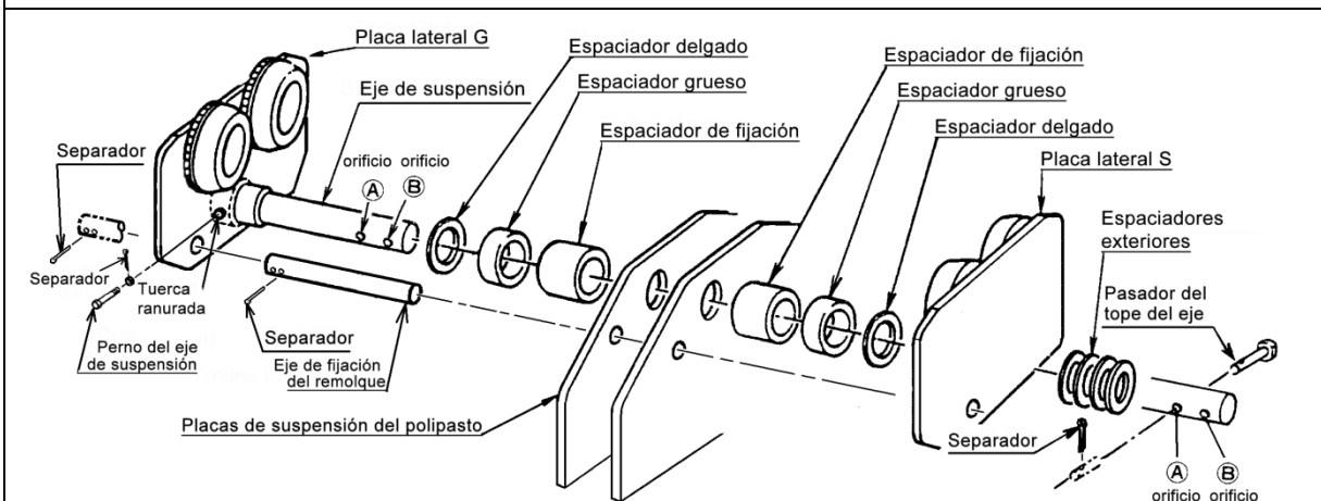
Figura 3-257 Ensamblaje del trole - Capacidades de 8 a 10 toneladas, CB o TCR
