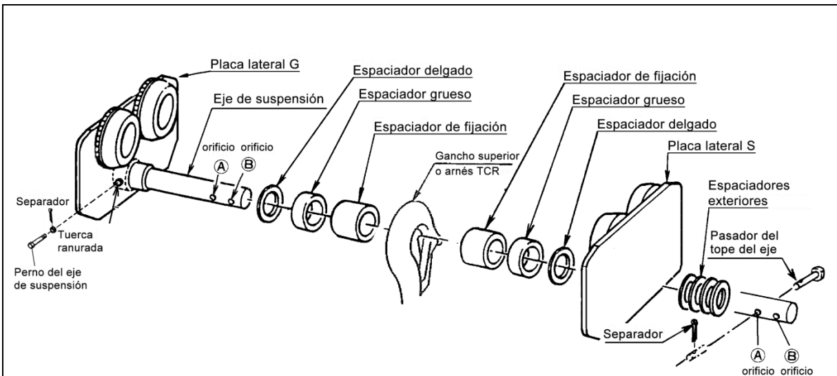
Figura 3-257 Ensamblaje del trole - Capacidades de 8 a 10 toneladas, CB o TCR
